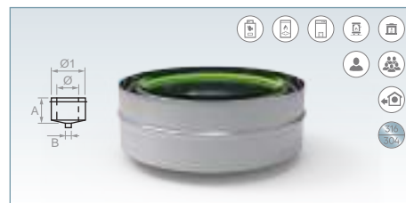
Tape con purga (Inox 316-Interior / Inox 304-Exterior)
