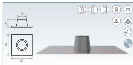
Teja plana (Inox 304)
