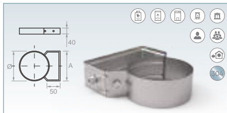
Soporte Mural (Inox 304)
