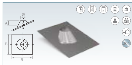
Teja inclinada 30° (Acero Inox 304)
